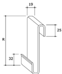
Gancho chato reto simples
