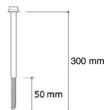
Parafuso com rosca soberba 8 x 300 mm
