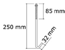
Gancho com rosca reto simples 8 x 250 mm com porca
