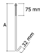
Gancho com rosca reto simples 8 mm com porca
