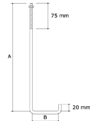
Gancho com rosca reto L
