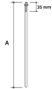
Pino com rosca
