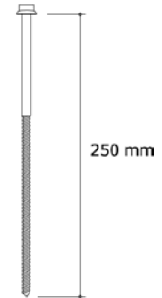
Parafuso com rosca soberba Ø 8 x 250 mm
