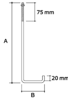
Gancho com rosca reto L
