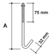
Gancho com rosca reto simples
