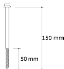
Parafuso com rosca soberba 8 x 150 mm
