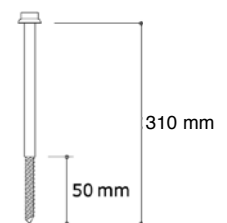
Parafuso com rosca soberba 8 x 310 mm
