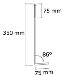
Gancho com rosca com uma extremidade 8 mm com porca
