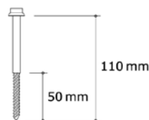
Parafuso com rosca soberba 8 x 110 mm
