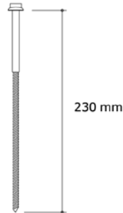
Parafuso com rosca soberba Ø 8 x 230 mm
