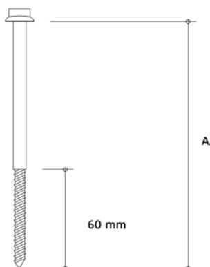
Parafuso com rosca soberba
