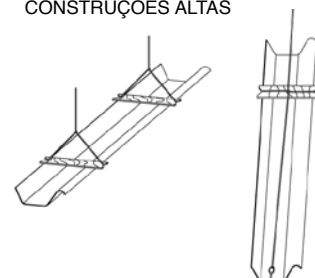
CONSTRUÇÕES ALTAS
