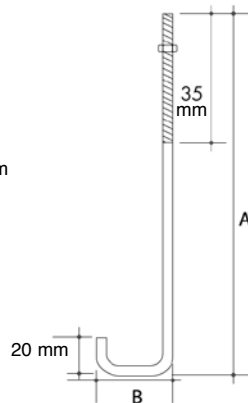
Gancho com rosca reto L
